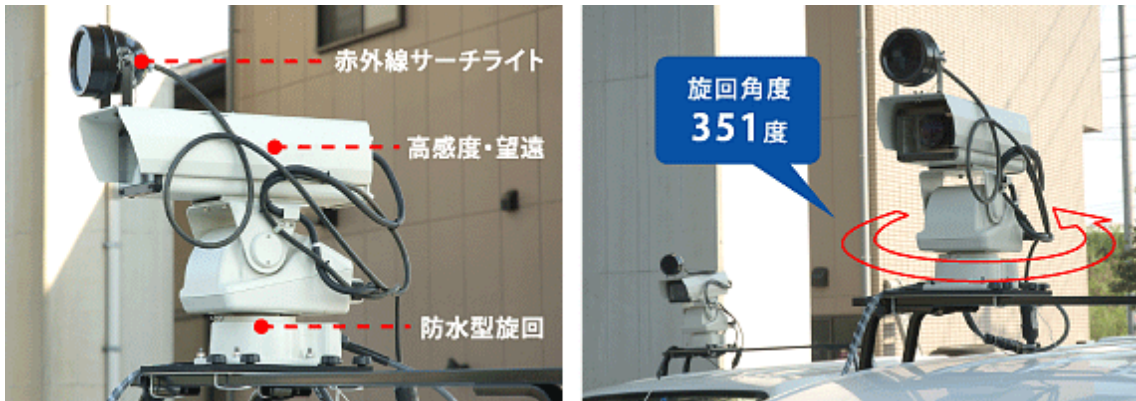
(写真3) 搭載した超高感度望遠暗視カメラ
