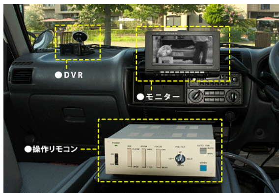
(写真5-1) 車内の録画機器
